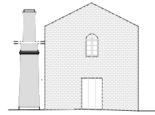
MILINO PROSPETTO EST
