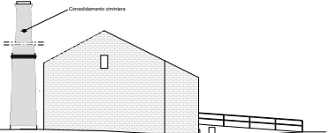
ESSICCATOIO PROSPETTO EST
